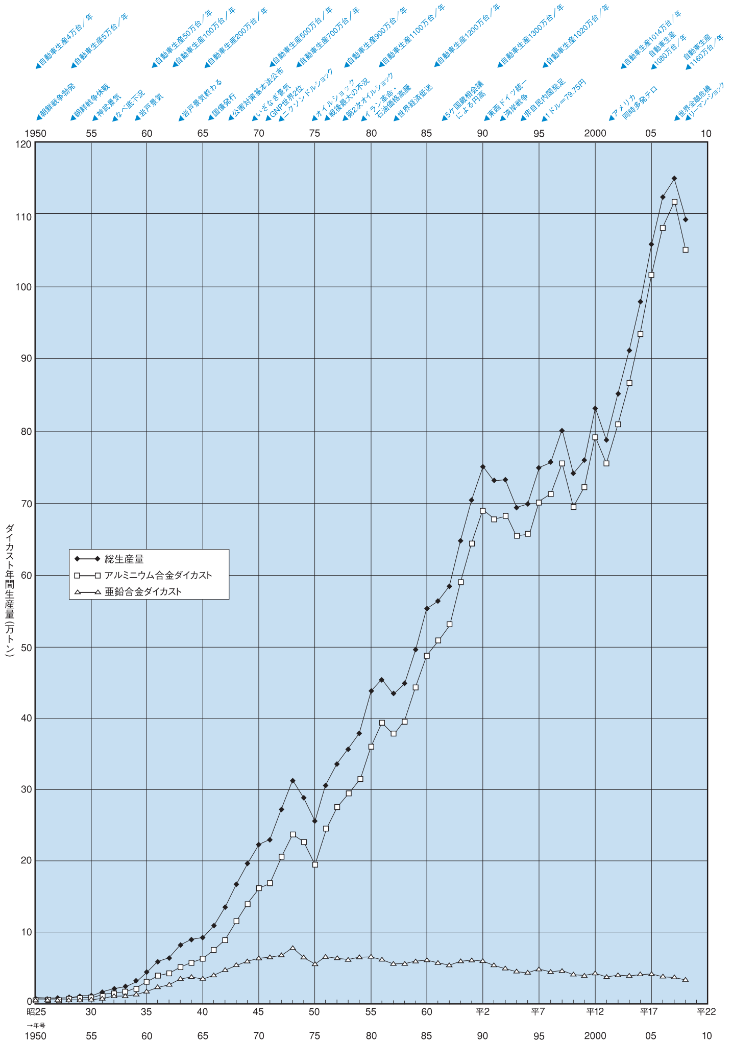
日本のダイカスト生産量(経済産業省/機械統計及び鉄鋼・非鉄金属・金属製品統計による)
